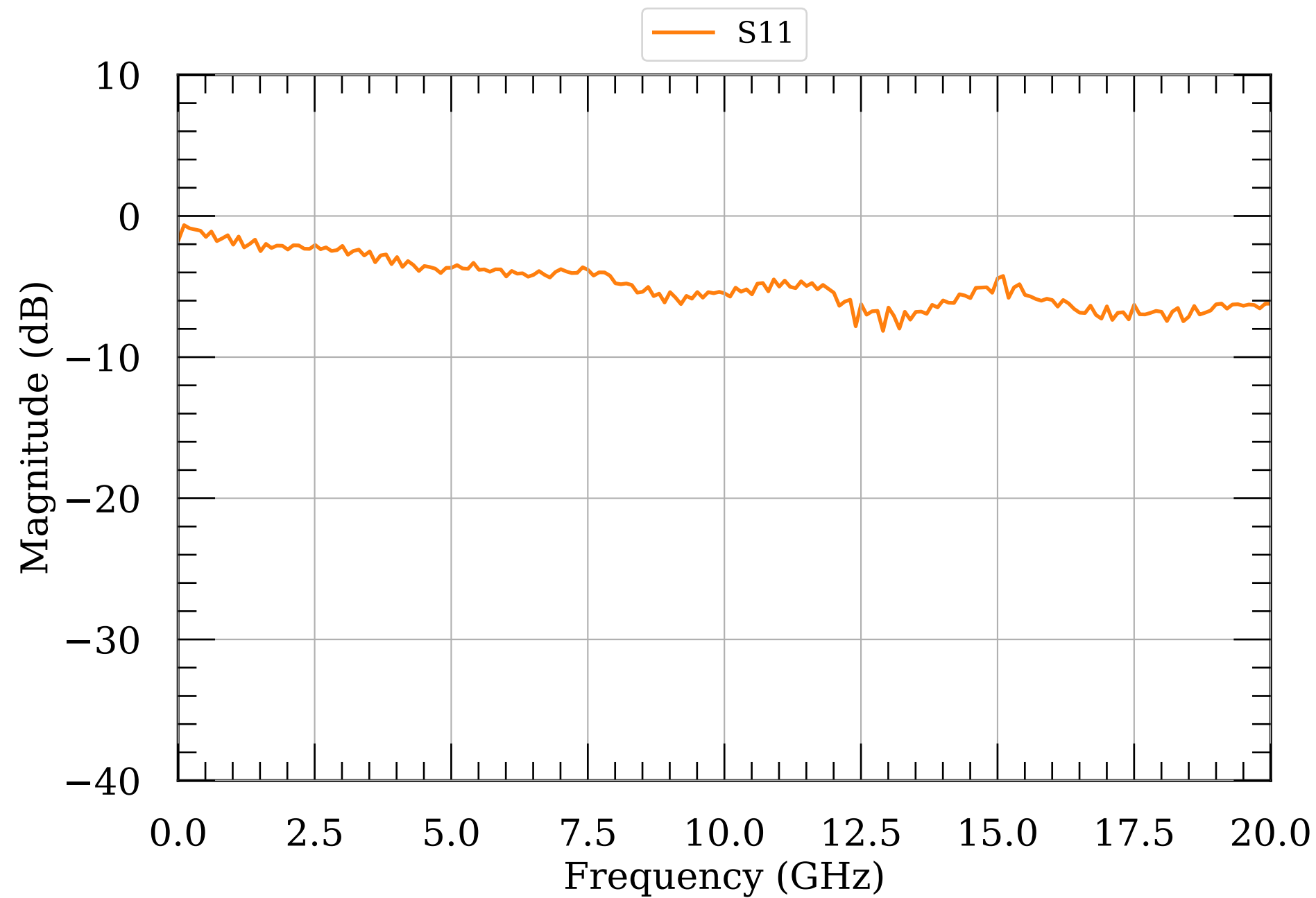
LNA S-params module087
